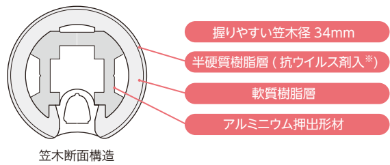
笠木断面構造
