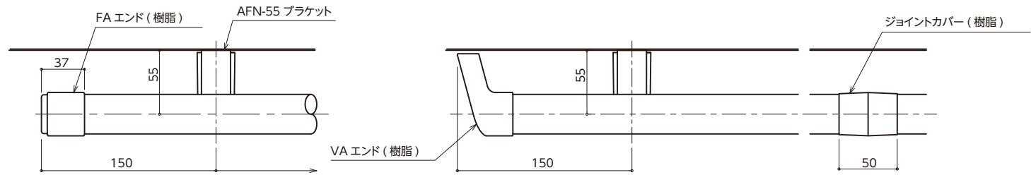
ストレートエンド平面詳細図
