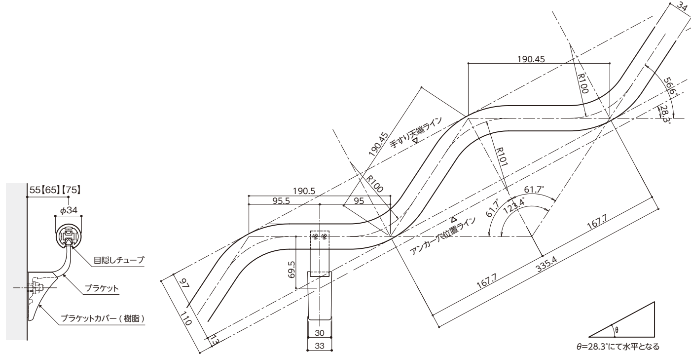
断面詳細図
