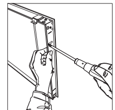
3 スライドアングル(2)の固定
